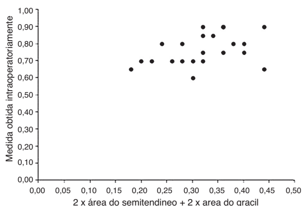
Figura 3 – Correlação entre a área calculada a partir do ultrassom (2 x área do semitendíneo + 2 x área do grácil) e a medida obtida intraoperatoriamente na amostra de 24 pacientes.
